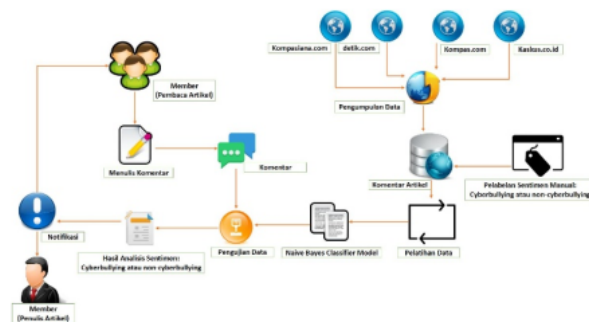
GAMBAR 2. Arsitektur Aplikasi Penyaring Komentar Cyberbullying
