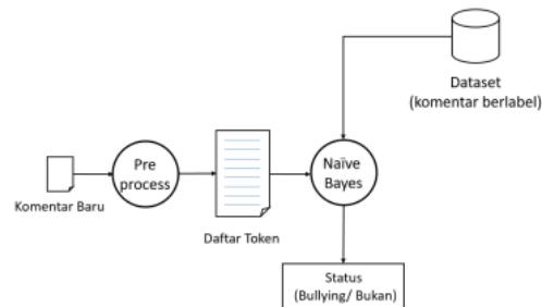
GAMBAR 3. Arsitektur Penyaring Komentar Cyberbullying
