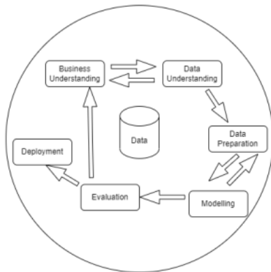
GAMBAR 2. Metodologi CRISP-DM
