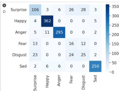
Gambar 6. Confusion Matrix K=1 dari hasil pengujian menggunakan google colab
