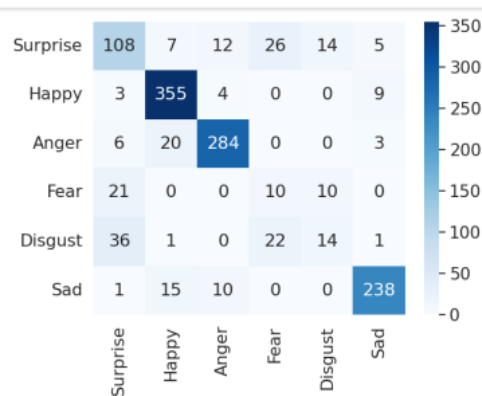
Gambar 10. Confusion Matrix K=5 dari hasil pengujian menggunakan google colab
