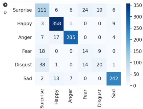
Gambar 8. Confusion Matrix K=3 dari hasil pengujian menggunakan google colab
