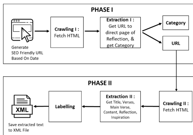
Gambar. 6. Rancangan Arsitektur Sistemrata
